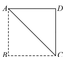
图5对折正方形 ABCD
