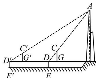
图6(测雕塑高)
