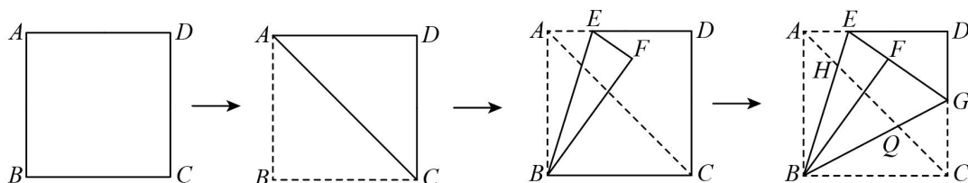
图4正方形 ABCD
